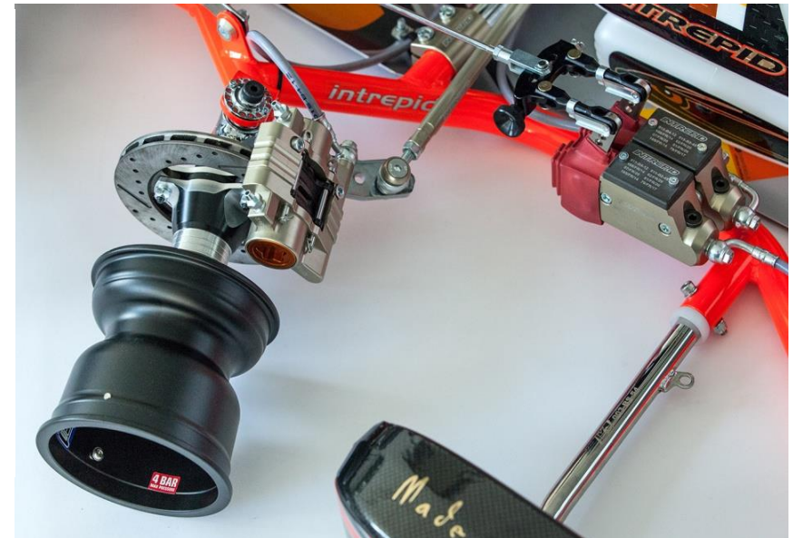
OPZIONAL WHELL SK1 (OPTIONAL)
